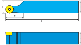
外徑車刀架 Tool holder
