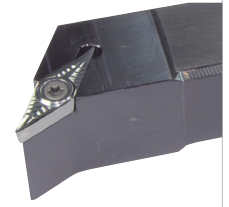
本圖所示為右手刀 (R)
